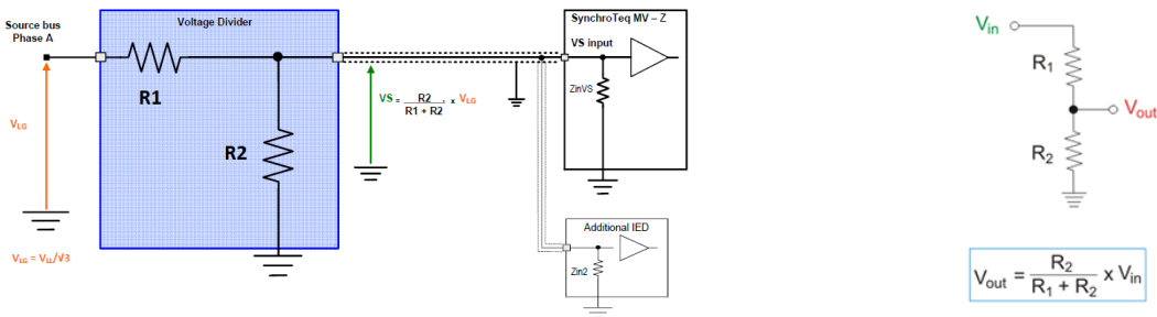
FIGURE 2 EXEMPLE DE DIVISEUR RÉSISTIF SUR L'ENTRÉE VS
