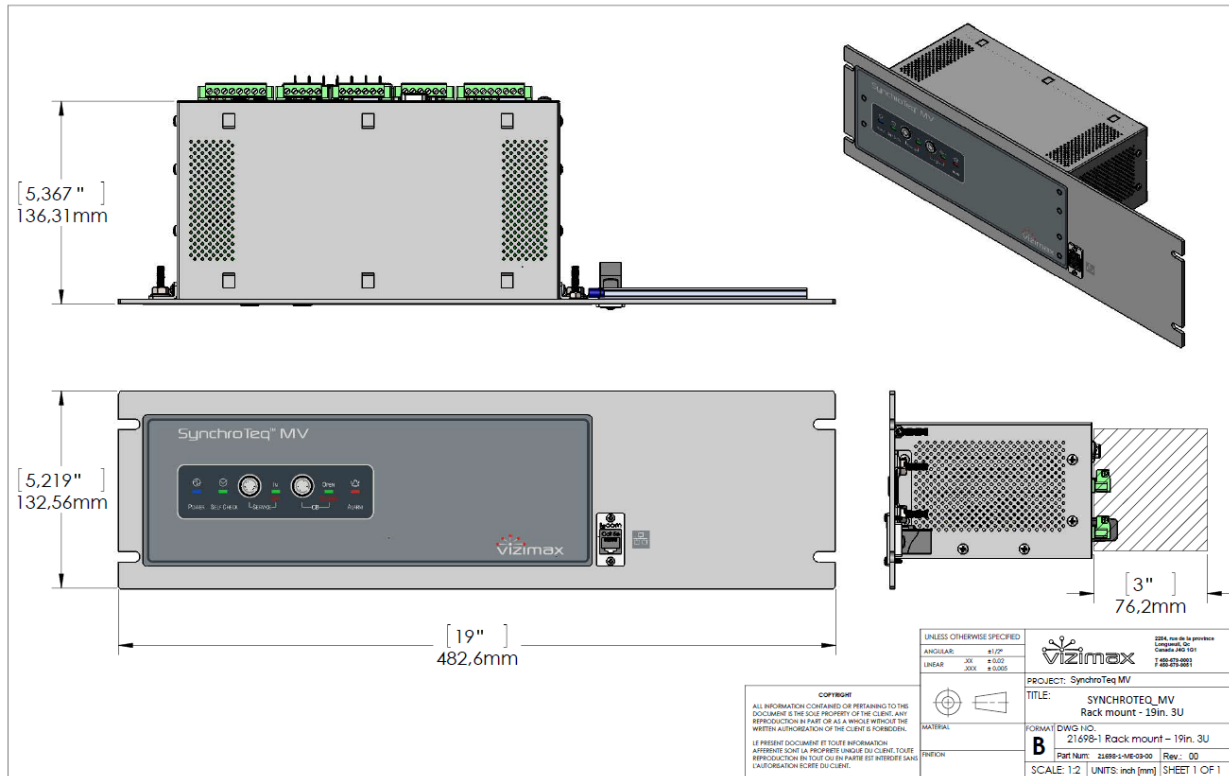
FIGURE 13 INSTALLATION EN RACK 19" (MODÈLE RM)
