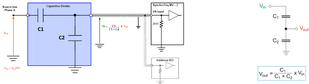
FIGURE 1 EXEMPLE DE DIVISEUR CAPACITIF SUR L'ENTRÉE VS
