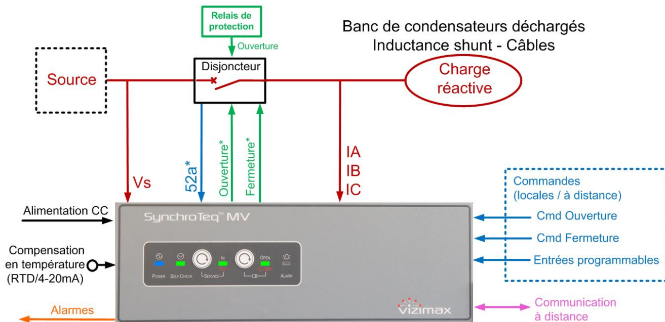
FIGURE 4 EXEMPLE DE SYNCHROTEQ MVR DANS UNE APPLICATION DE CHARGE RÉACTIVE DÉCHARGÉE
