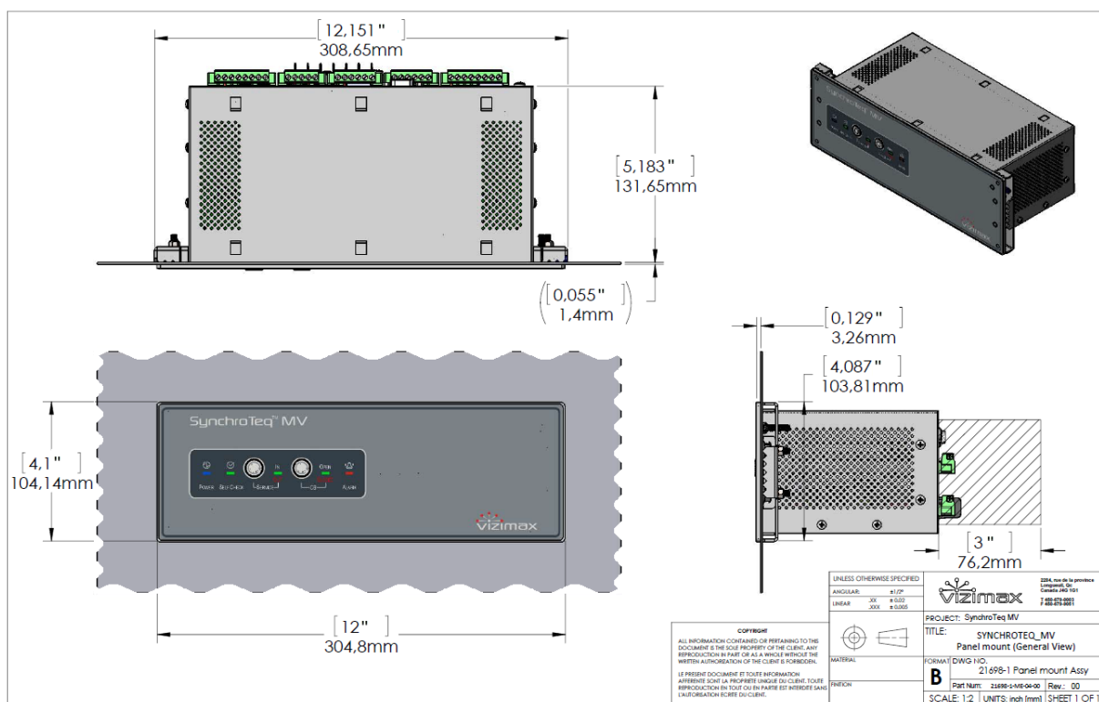
FIGURE 12 INSTALLATION SUR PANNEAU
