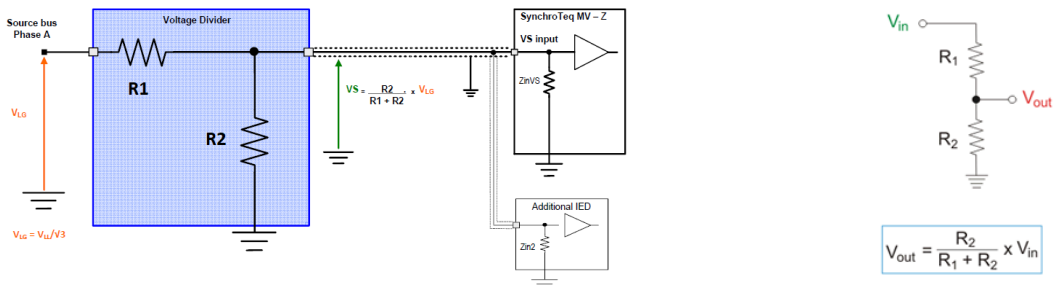
FIGURE 2 EXEMPLE DE DIVISEUR RÉISTIF SUR L'ENTRÉE VS
